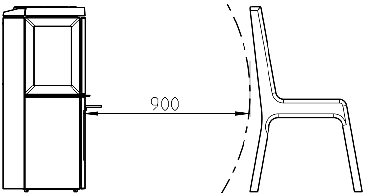
Min. avstand til møbler / brennbart materiale:
